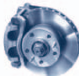
Dvoukruhový brzdový systém je vybaven kotoučovými brzdami na všech kolech. Přední kotouče o průměru 280 až 300 mm jsou ventilované.
